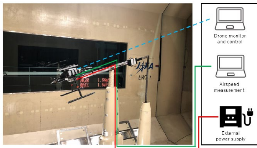
図3 実験のセットアップ（左：風洞内部、右：風洞外側）
