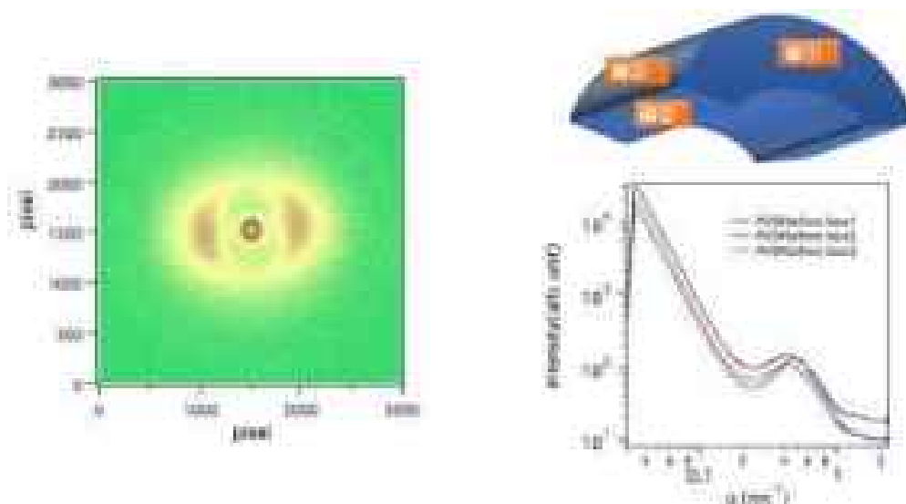
図 16 (左)レーザー光散乱による異方性観察結果；(右上)PVDF 円筒形試料における切り出し面①～③；(右下)①～③における X 線小角散乱の実験結果
