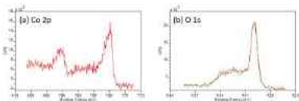
図 8 6 keV 励起で測定した CoO 粉末の HAXPES スペクトル。(a) Co 2p (b) O 1s
