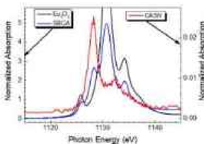
図 9 部分蛍光法で取得した \text{Eu}_2\text{O}_3 と 2 種類の Eu 蛍光体の Eu M_5 吸収スペクトル
